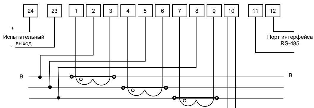
Рисунок В.4 – Схема подключения счетчика ЭЭ8005-К трансформаторного включения
