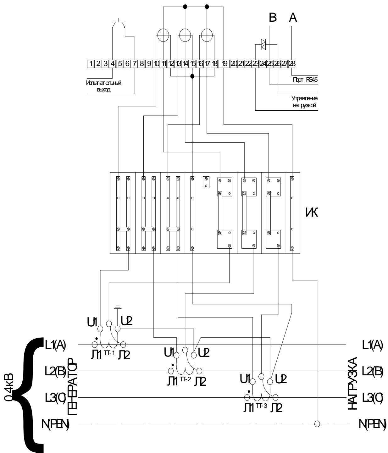
Рисунок В.5 – Восьмипроводная схема подключения счетчика трансформаторного включения с испытательной колодкой
