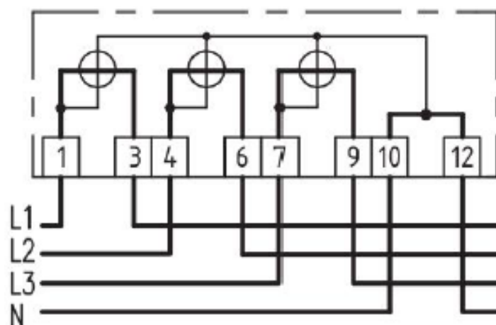
Рисунок Б.1 – Схема подключения счетчика непосредственного включения в трехфазную четырехпроводную сеть напряжением 0,4 кВ
