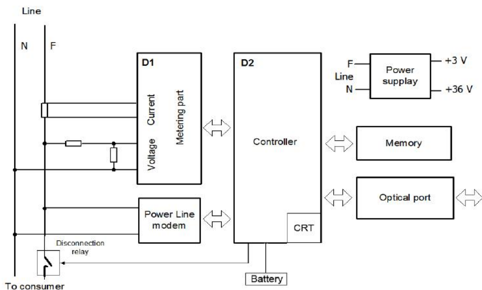
Рис. 2.1 Блок-схема счётчика в полной комплектации (а) и столбового счётчика (b)
